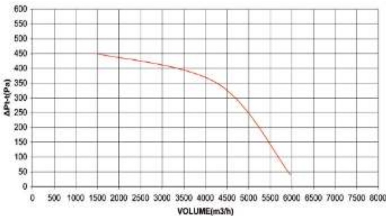
Ø250-1.5HP-1450RPM
